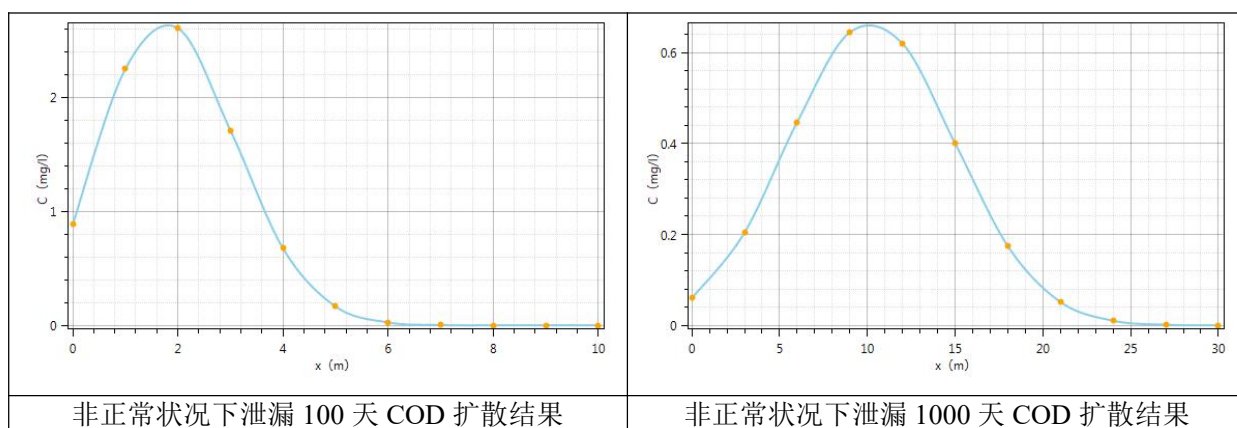
图 5.2-14 非正常状况下污染物扩散结果
