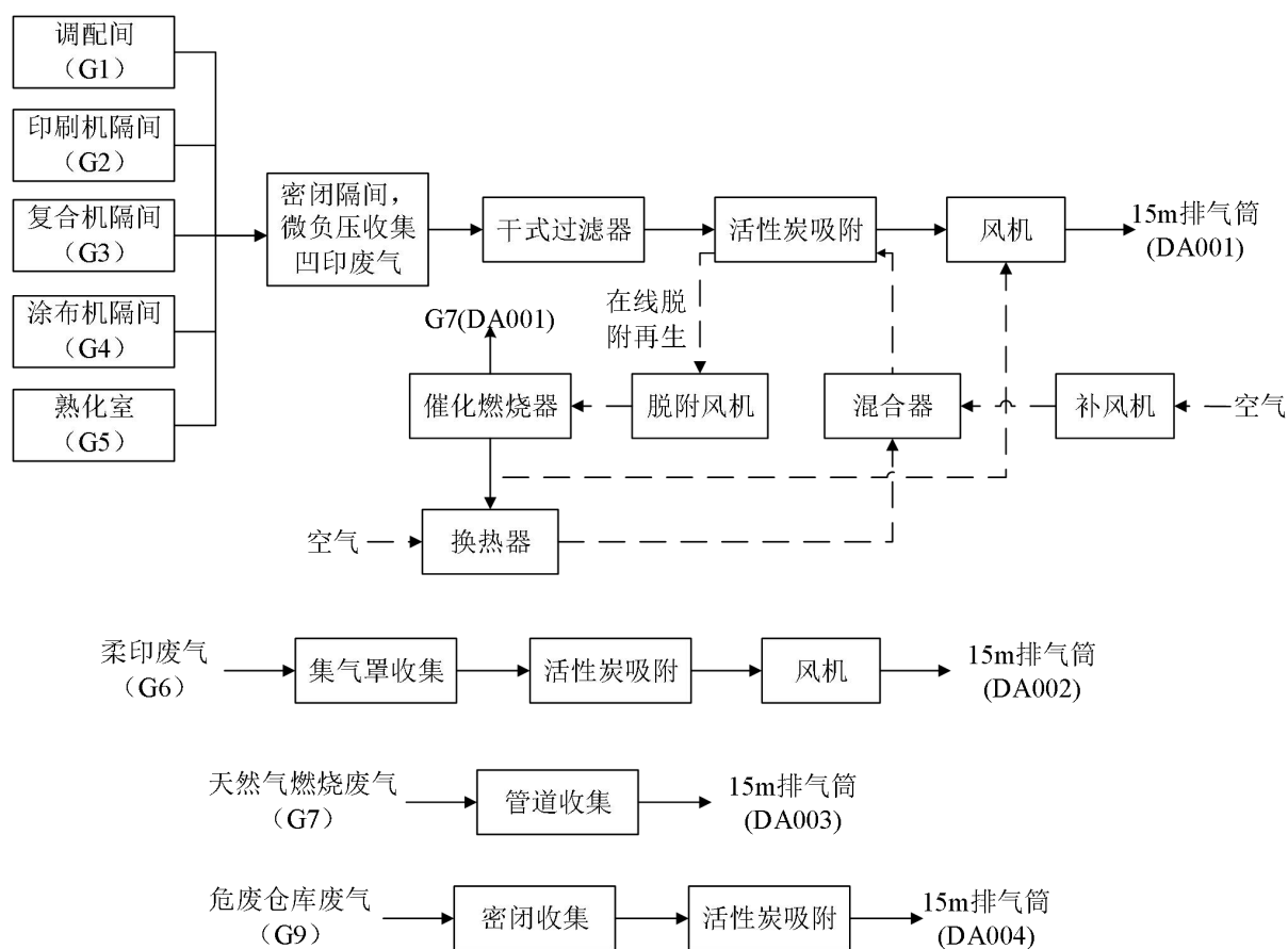
图 6.1-1 项目废气污染防治措施汇总图
