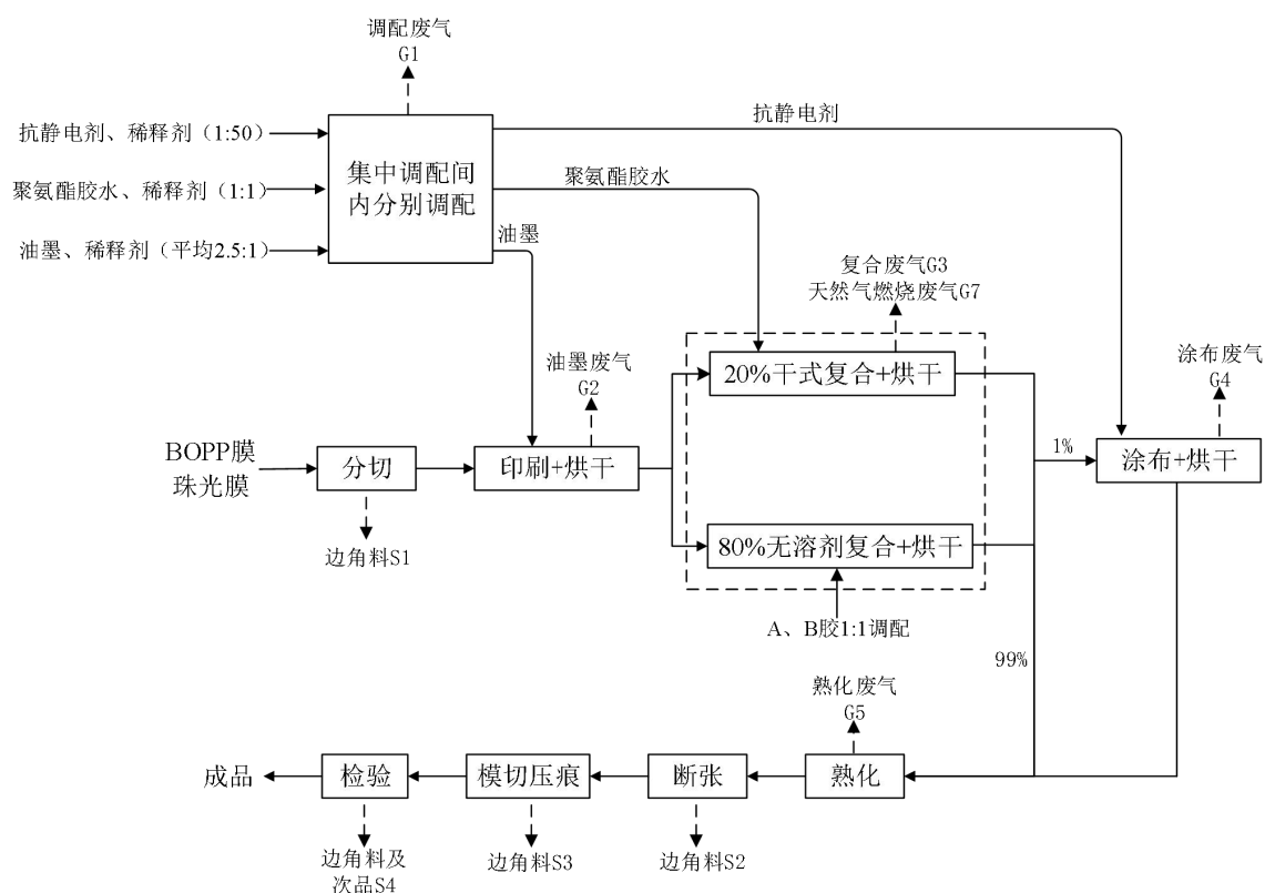
图 3.2-1 凹印标签生产工艺流程及产污环节图
